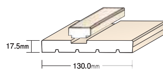
在来用内部ドア枠
