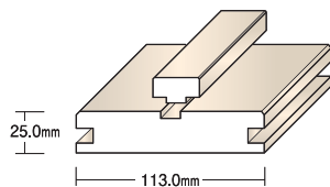
差込型内部ドア枠
