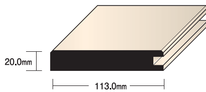
サッシ枠 RC602-39 \ell = 3900 \text{ mm} ¥10,400
