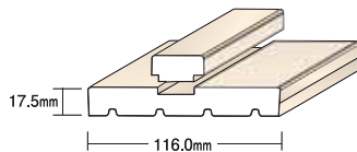
2×4用内部ドア枠
