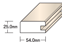
片引き戸用 中方立
