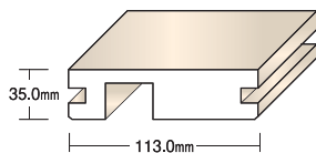
片引き戸用上部枠
