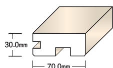
折戸用上レール (別途)
