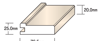
片引き戸用 戸当
