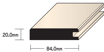
サッシ枠 RC601-39 \ell = 3900 \text{ mm} ¥7,700
