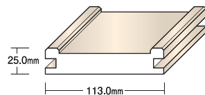
引き戸用縦枠(左右兼用)
