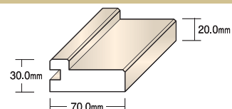
折戸用上レール (別途)
