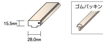
戸当(パッキン付き) RC061T-21
