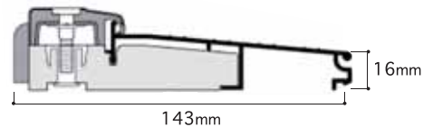
【内開き用】
